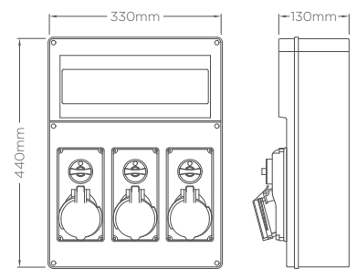
RE119F Enclosure
